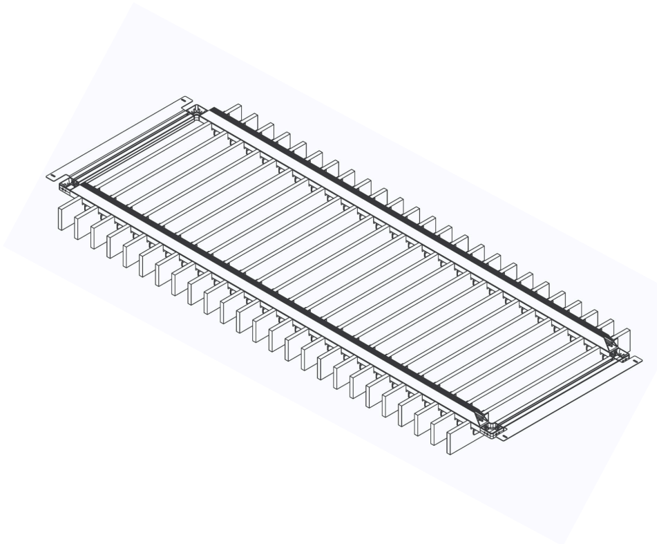
BMGCON-C02 Auvent intermédiaire 2,45 m
