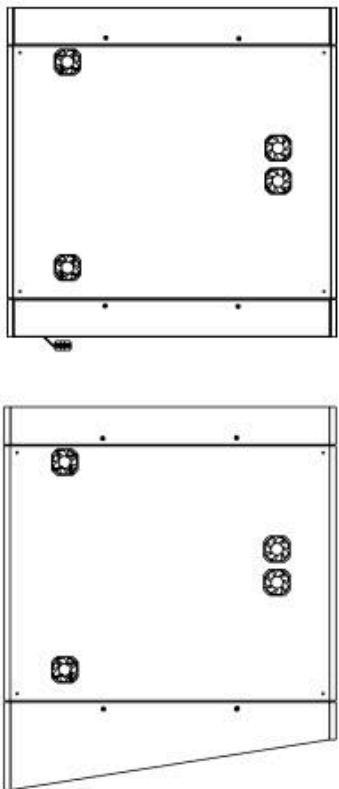
Vue en plan 4 ventilateurs. Haut : sans kink Bas : avec kink
